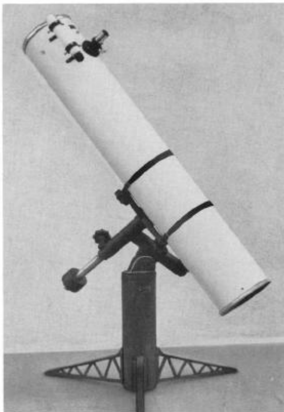
8" F/7 STANDARD
